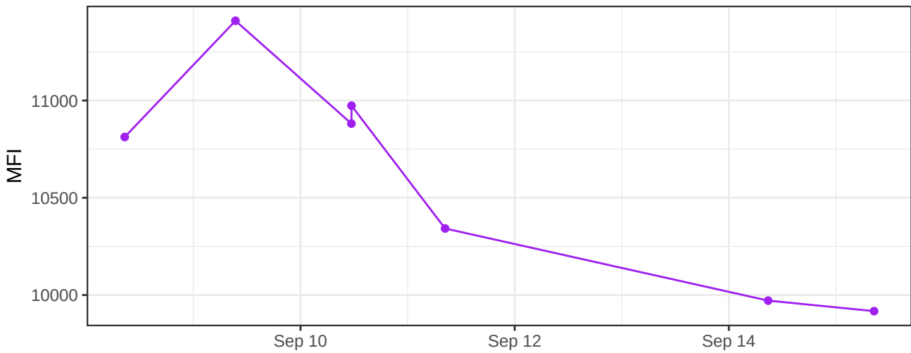
UV515-A
