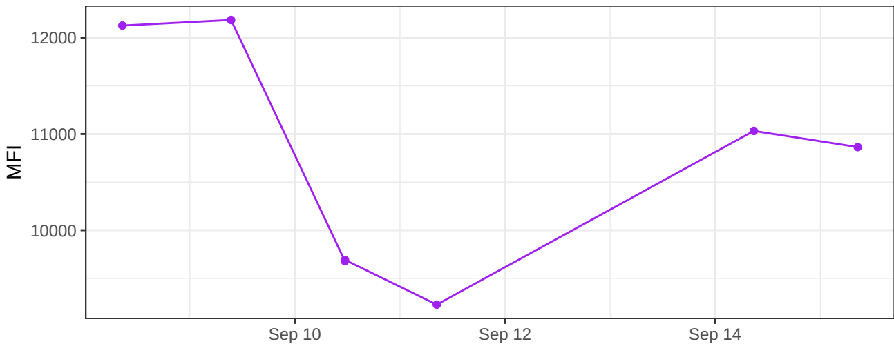
UV446-A
