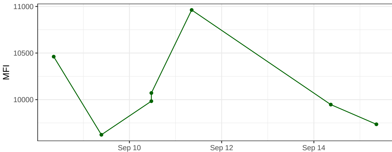
YG602-A
