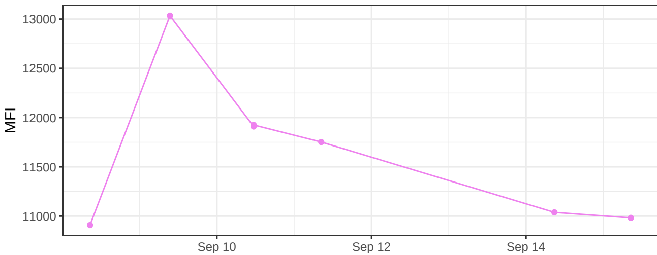
V785-A
