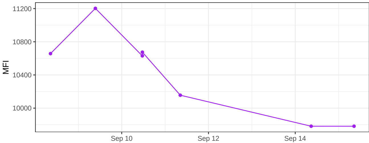
UV515-A
